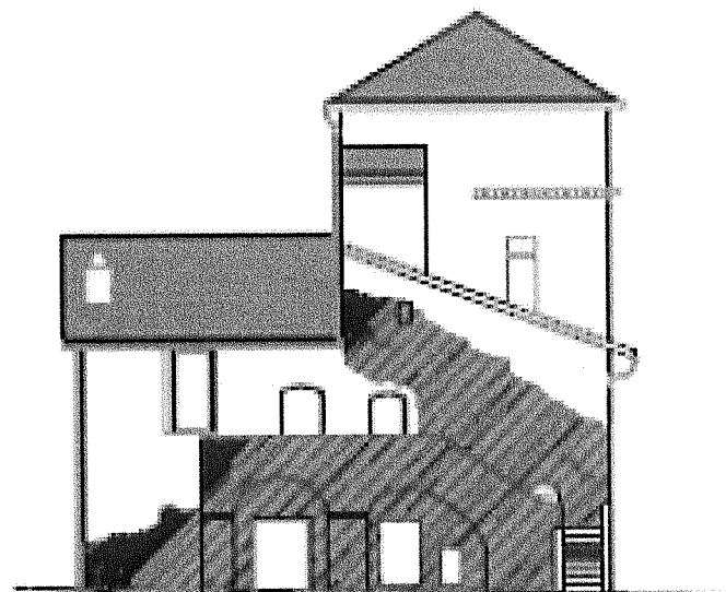
PROSPETTO OVEST
